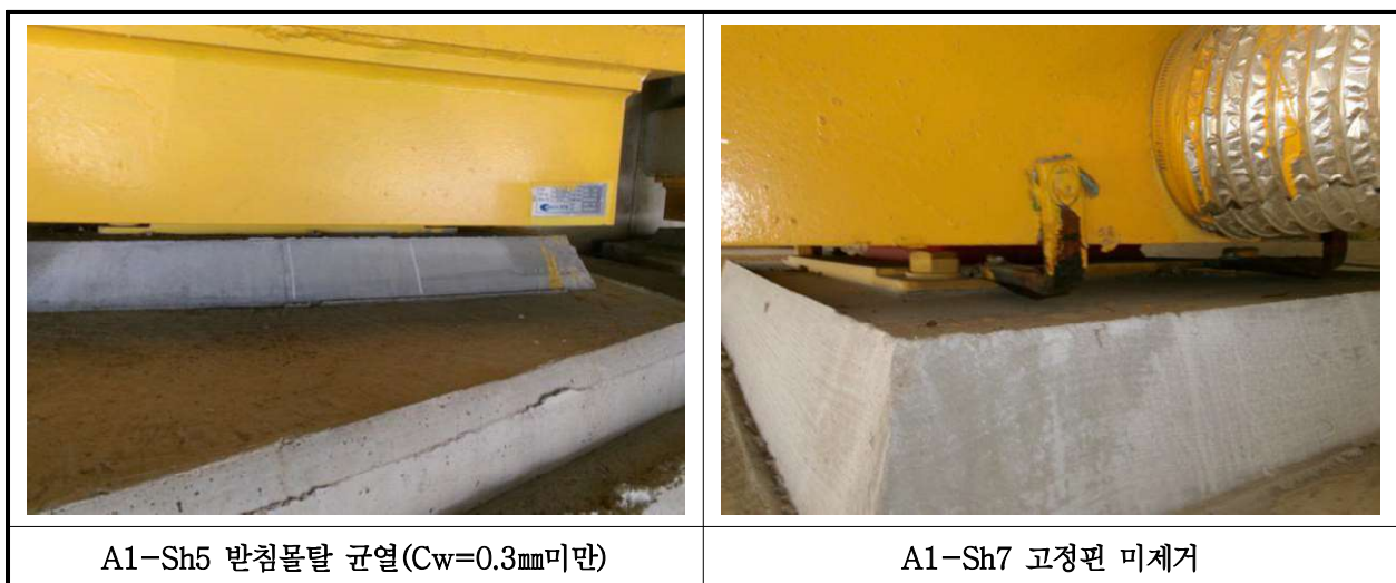
【사진 19.3.13】 교량반침 손상현황
