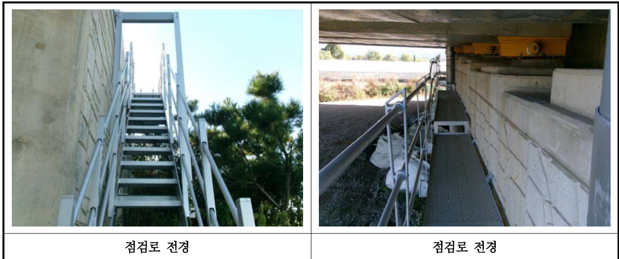
【사진 19.3.25】 교량 점검시설 전경
